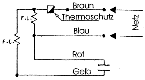
Anschlußschema
